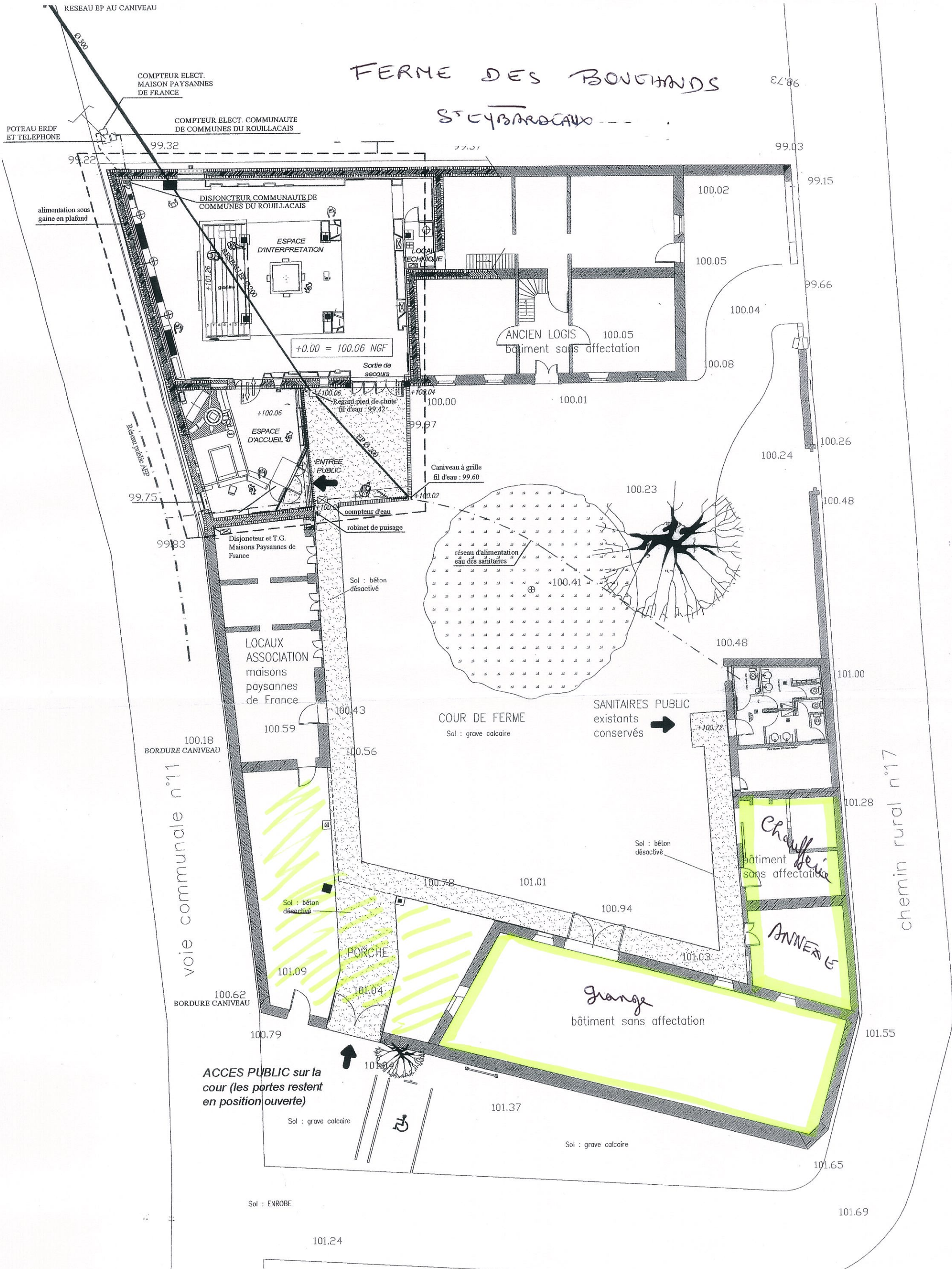
PLAN NIVEAU RDC COTES ALTIMETRIQUES RATTACHEES AU NGF
